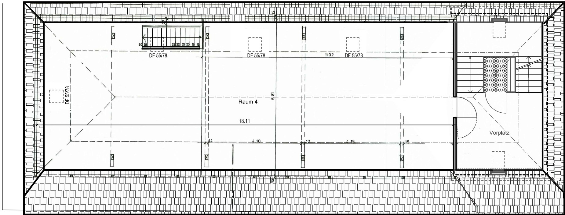
Dachgeschoss
